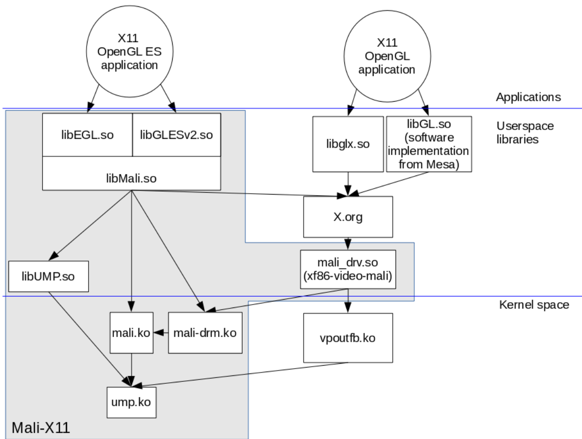
Рисунок 2.1. Диаграмма зависимостей OpenGL и OpenGL ES-приложений X11
