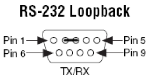
Рисунок 3.1. Включение режима loopback порта RS232 на модулях Салют-ЭЛ24Д1 r1.3, r1.4, Салют-ЭЛ24Д2 r1.1
