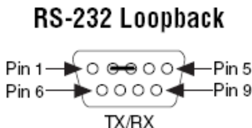
Рисунок 3.1. Включение режима loopback порта RS232 на модулях Салют-ЭЛ24Д1
