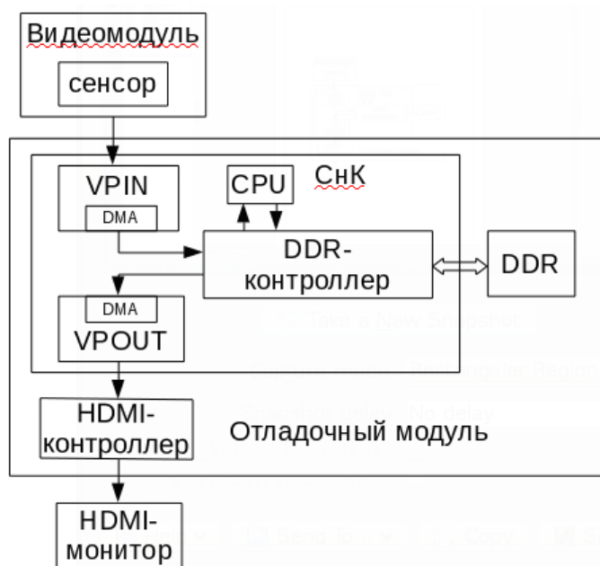
Рисунок 3.2. Диаграмма потоков видеокадров
