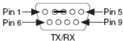
Рисунок 3.1. Включение режима loopback порта RS232 на модулях Салют-ЭЛ24Д1 r1.3, r1.4, Салют-ЭЛ24Д2 r1.1
