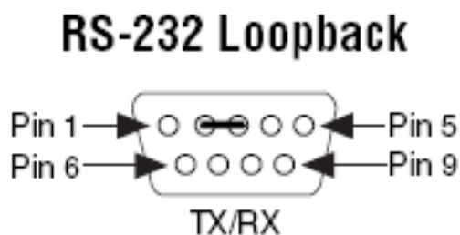
Рисунок 3.1. Включение режима loopback порта RS232 на модулях Салют-ЭЛ24Д1 r1.3, r1.4, r1.5
