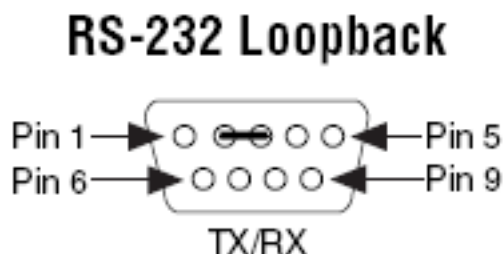
Рисунок 3.1. Включение режима loopback порта RS232 на модулях Салют-ЭЛ24Д1 r1.3, r1.4, r1.5
