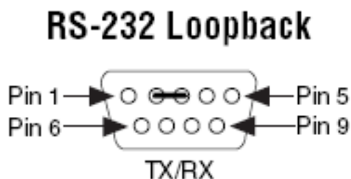
Рисунок 3.1. Включение режима loopback порта RS232 на модулях Салют-ЭЛ24Д1
