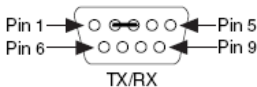
Рисунок 3.1. Включение режима loopback порта RS-232 на модулях Салют-ЭЛ24Д1
