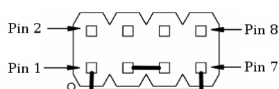
Рисунок 3.3. Включение режима loopback порта RS-485 на модуле Салют-ЭЛ24Д2
