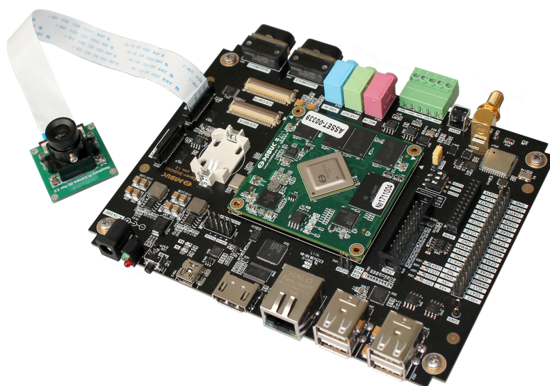
Рисунок 3.2. Пример подключения видеомодуля RPi Camera (B) к модулю Салют-ЭЛ24ОМ1 r1.2
